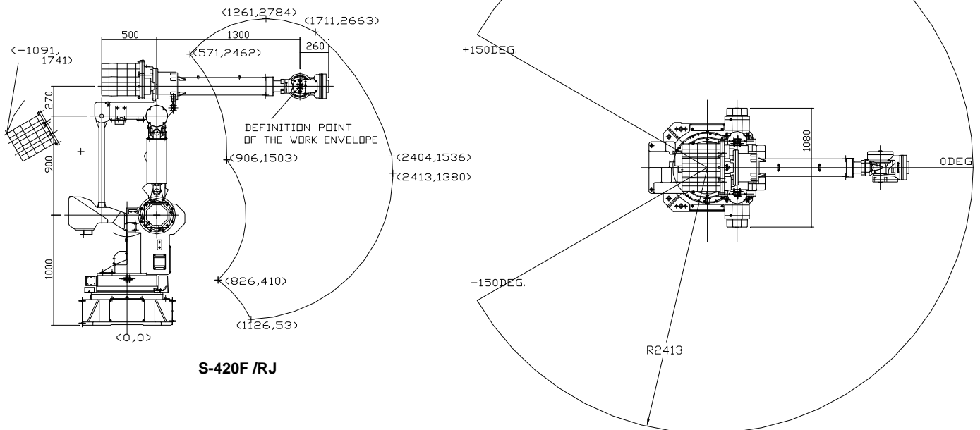
Maßskizze eines S-420-RJ Roboters, diese ist weitgehend maßlich identisch mit dem RH-Modell
